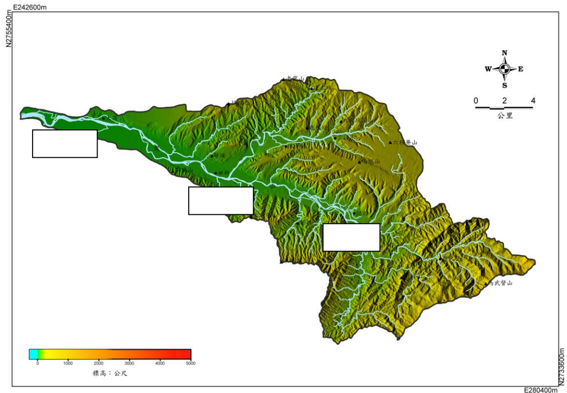
圖 2-4 鳳山溪流域水系彩繪明暗圖
